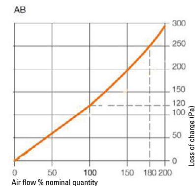
CURVA CARATTERISTICA DEL FILTRO
