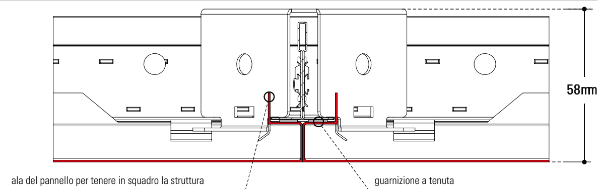
sezione di due pannelli affiancati
